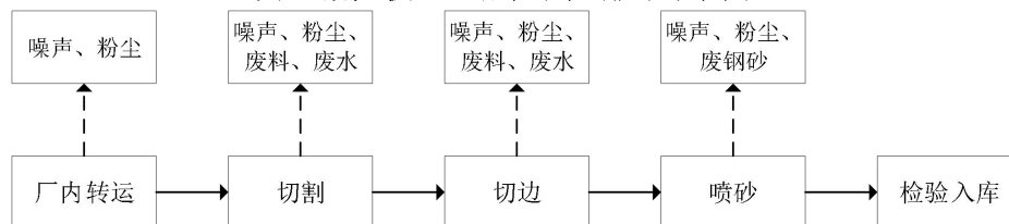
图 3 喷砂板工艺流程和产排污环节图
