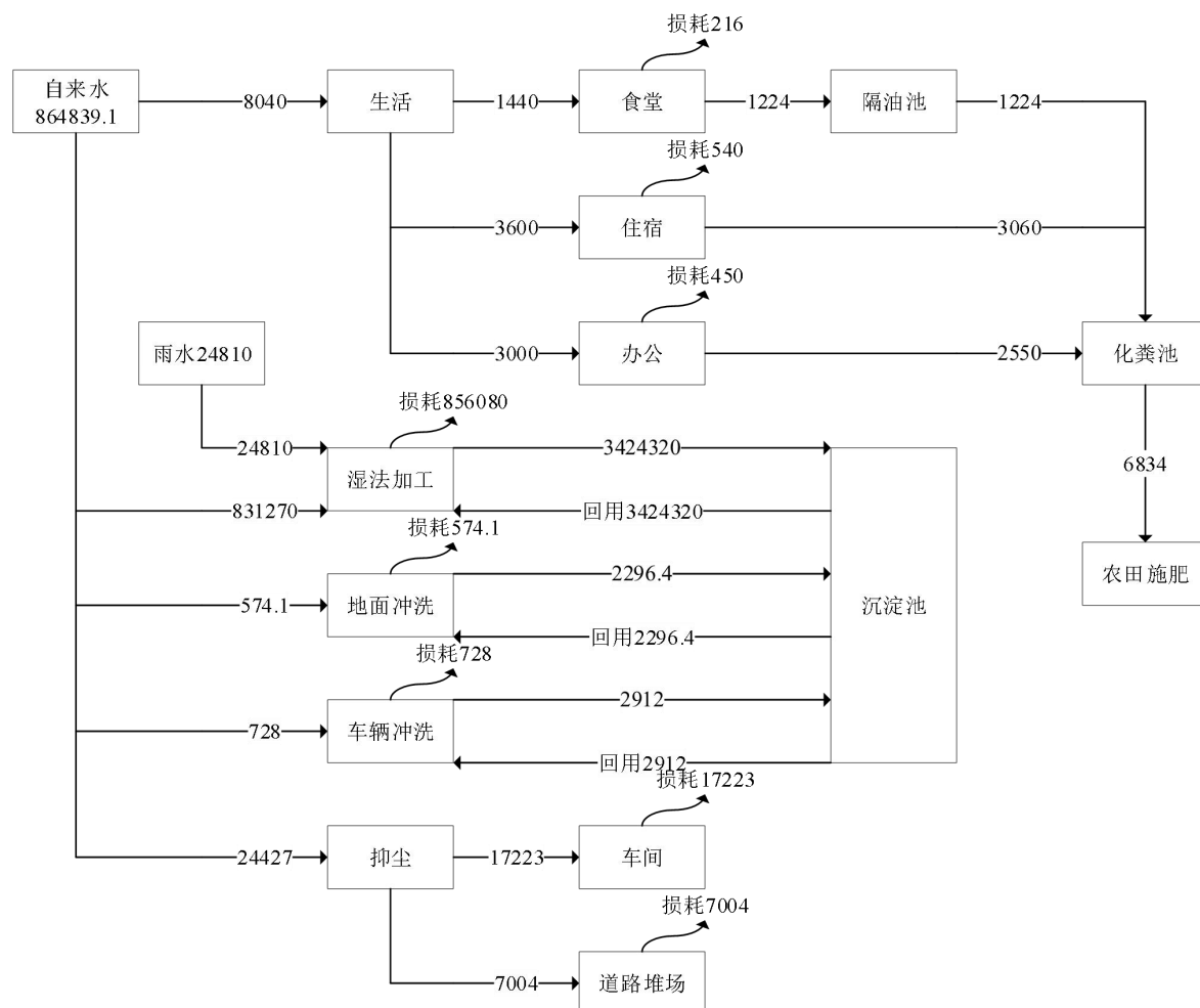
图 1 项目水平衡图 (单位: \text{m}^3/\text{a} )
