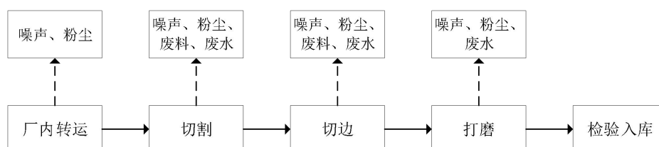
图 2 磨光板工艺流程和产排污环节图
