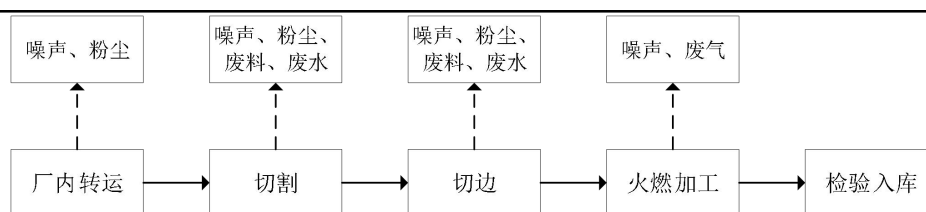
图 4 火烧板工艺流程和产排污环节图
