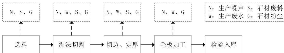
图5 毛板生产工艺流程及产污节点图
