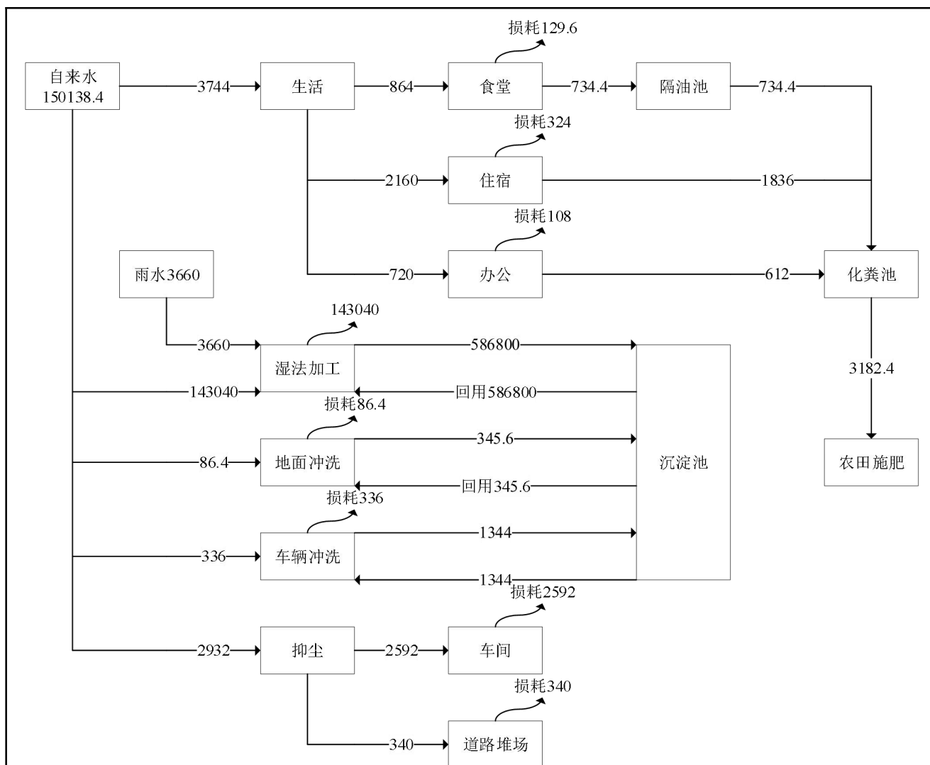
图1 项目水平衡图 (单位: m³/a)
