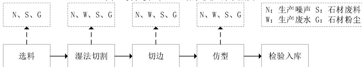
图7 路沿石、异型材生产工艺流程及产污节点图
