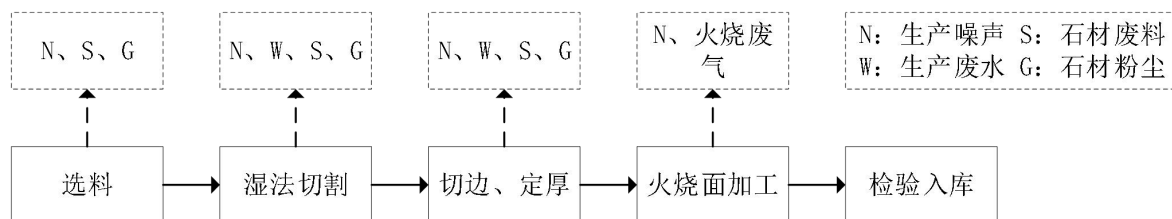
图2 火烧板生产工艺流程及产污节点图
