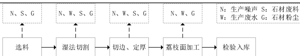
图4 荔枝板生产工艺流程及产污节点图
