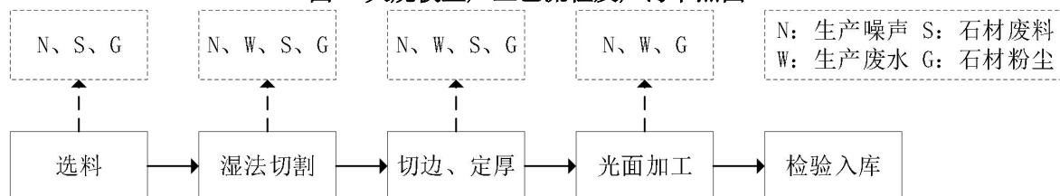
图3 磨光板生产工艺流程及产污节点图
