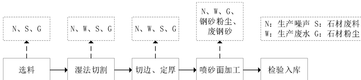
图6 喷砂板生产工艺流程及产污节点图
