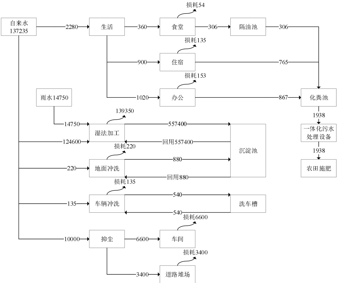
图 1 项目水平衡图（单位：m³/a）
