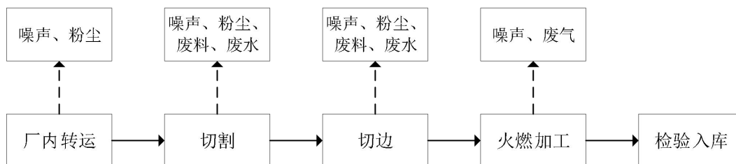
图 3 火烧板工艺流程和产排污环节图
