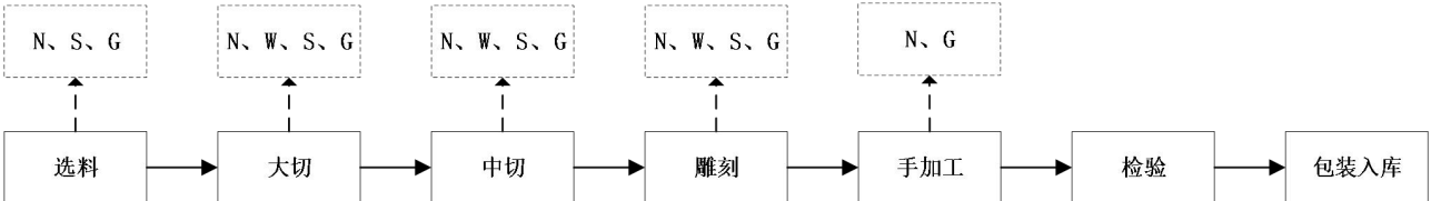
图3 雕刻板生产工艺流程及产污节点图
