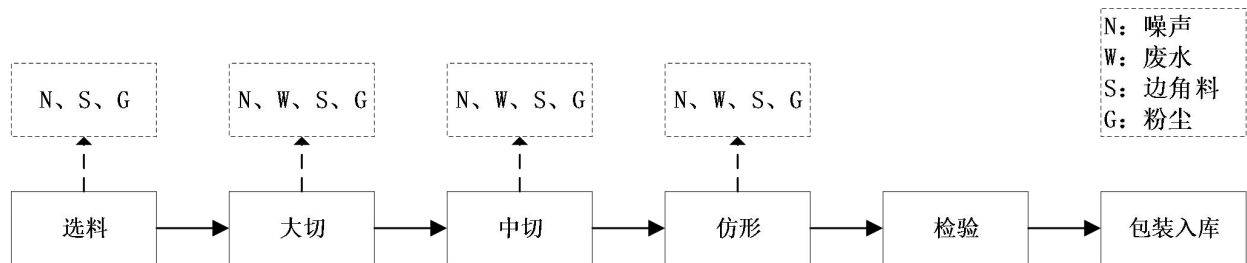
图2 路沿石生产工艺流程及产污节点图
