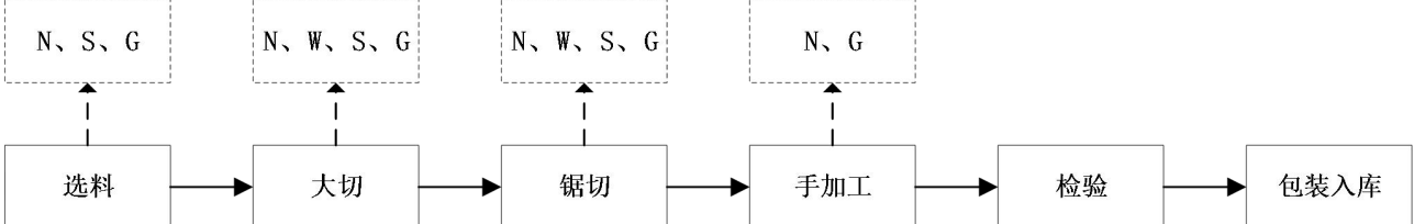
图4 圆柱材生产工艺流程及产污节点图
