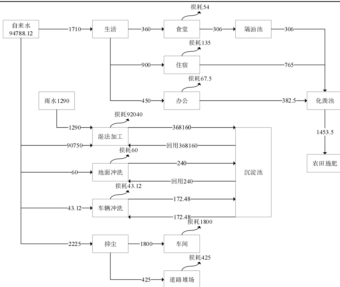
图 1 本项目阶段验收全厂水平衡图（单位：m³/a）
