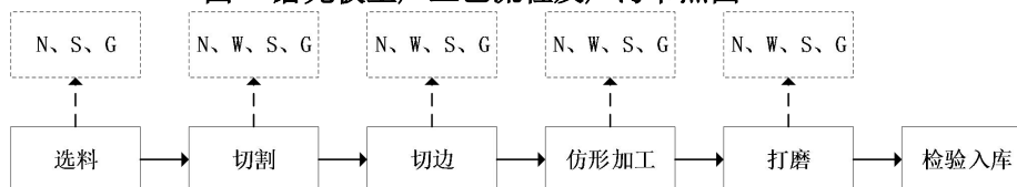
图5 路沿石生产工艺流程及产污节点图
