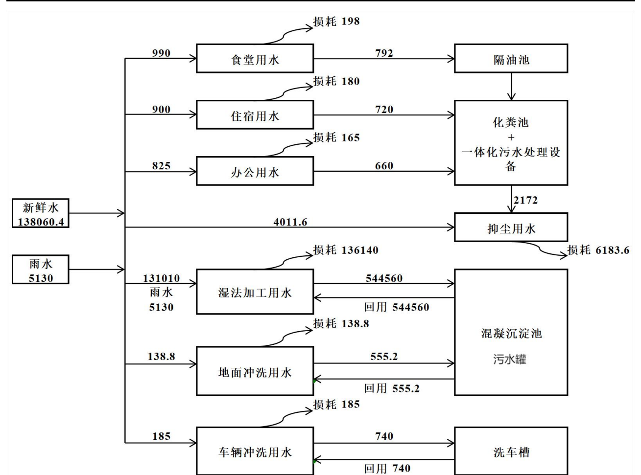
图 1 项目水平衡图 (单位: m³/a)
