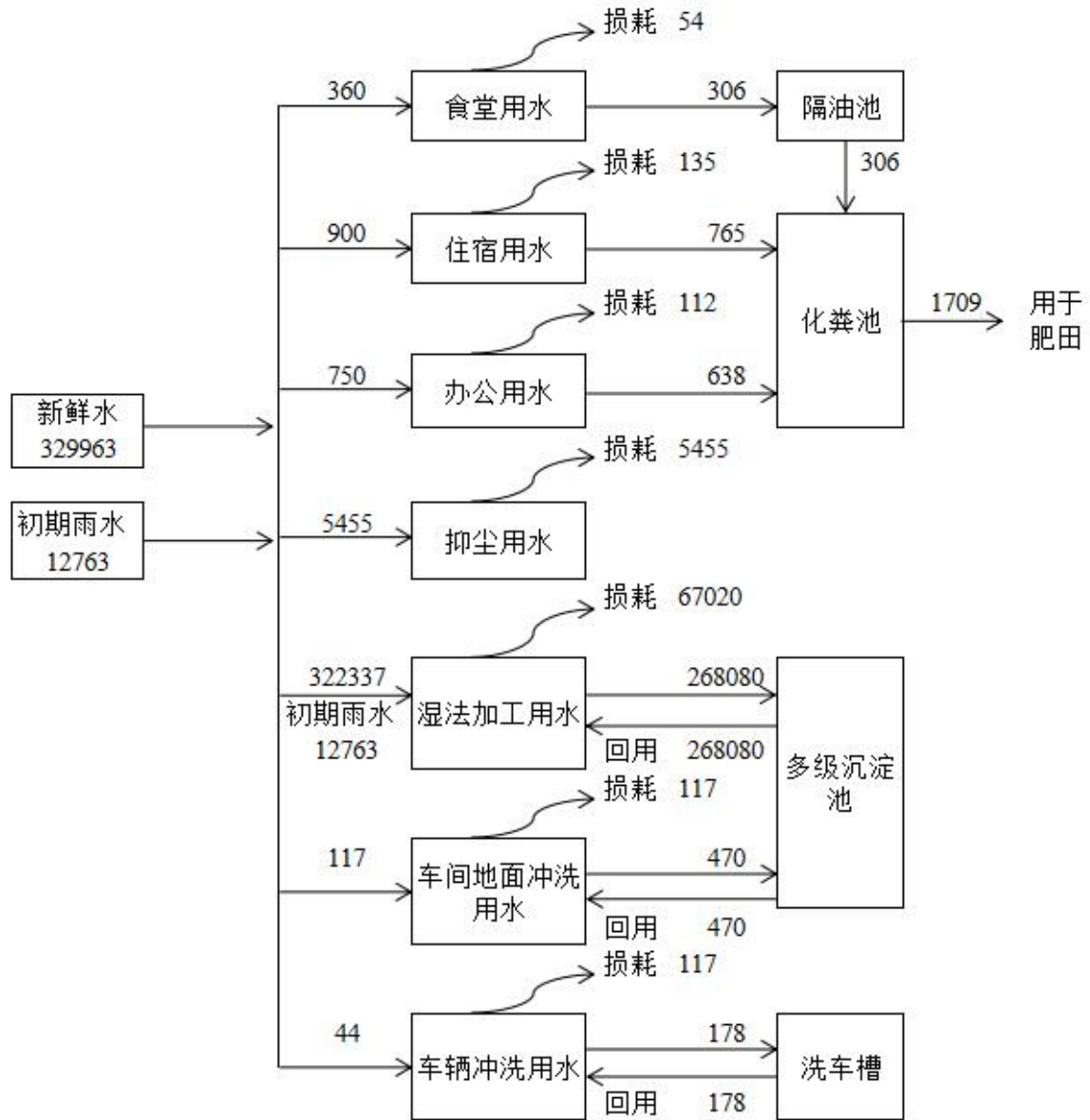
图 1 项目水平衡示意图 (单位: \text{m}^3/\text{a} )
