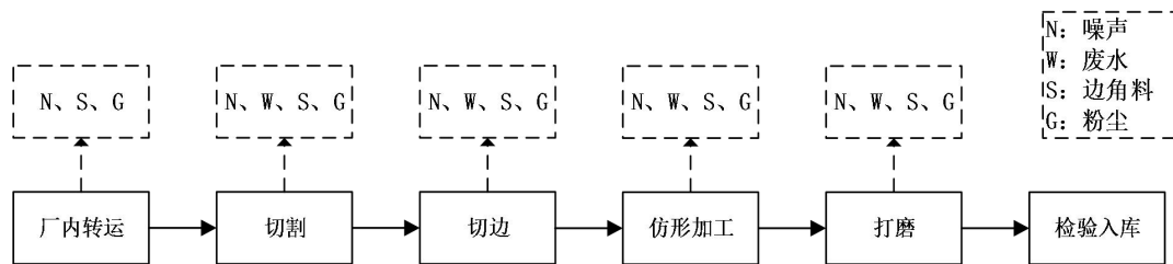
图4 路沿石生产工艺流程及产污节点图
