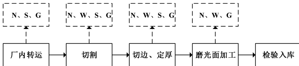
图3 磨光板生产工艺流程及产污节点图
