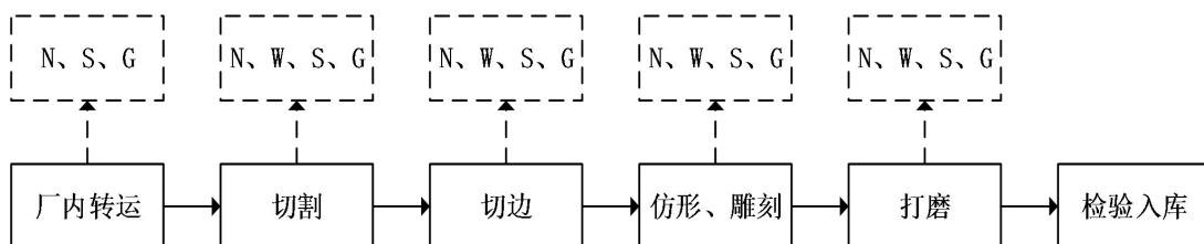
图5 其他仿形雕刻板材生产工艺流程及产污节点图
