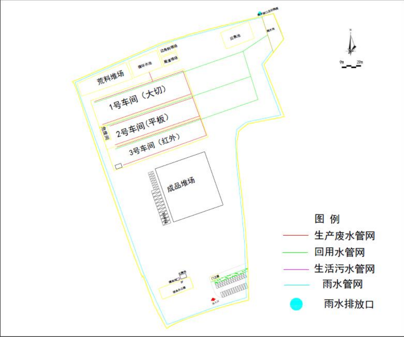
附图三 平面布置图
