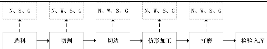
图4 路沿石生产工艺流程及产污节点图
