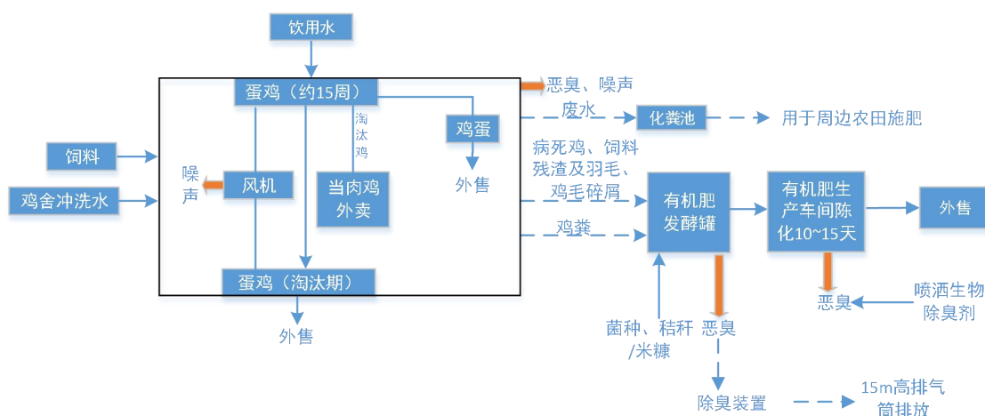
图2 蛋鸡饲养环节及产污节点图
