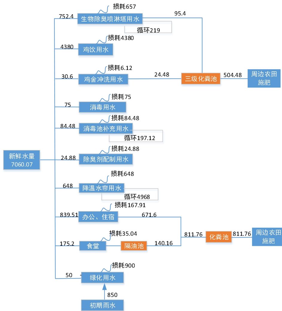
图 1 验收阶段本项目水平衡图（单位： \text{m}^3/\text{a} ）
